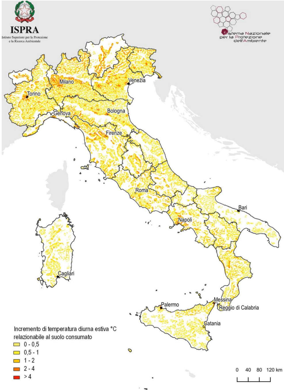
Figura 93. Incremento di temperatura (LST) media diurna estiva (°C) per gli anni dal 2017 al 2019, relazionabile alla densità di suolo consumato. Fonte: elaborazioni ISPRA su cartografia SNPA e dati MODIS
